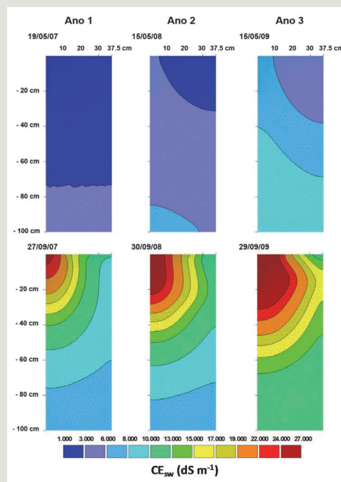
Figura 4 – Simulação da distribuição da condutividade eléctrica da solução do solo ( \text{CE}_{\text{sw}} ) num perfil de solo regado com águas salinas, durante 3 ciclos culturais, à data da sementeira (parte superior) e da colheita (parte inferior). O gotejador localizava-se no canto superior esquerdo de cada perfil de solo apresentado. Fonte: Ramos et al. (2012)
